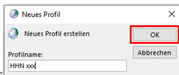
Fig. 2: Fenster „Mail-Setup“
