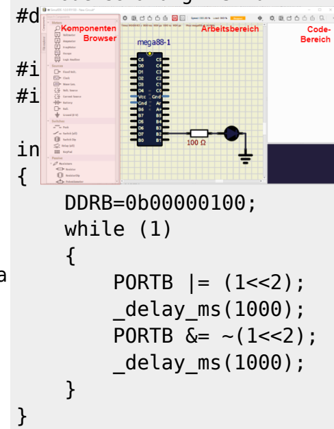
Fig. 1: einfache Diodenschaltung in SimulIDE
