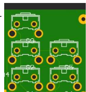
Fig. 2: Beispiel für schlechte Anordnung für ein seitlich-bediensbares
