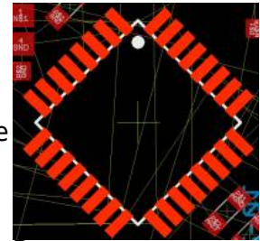
C Beispiel für besseres Airwiring
