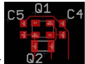
D Beispiel für Bauteilgruppe Quarz
