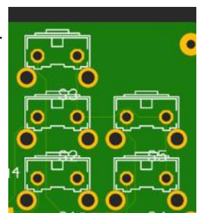
Fig. 2: Beispiel für schlechte Anordnung für ein seitlich-bediensbare
