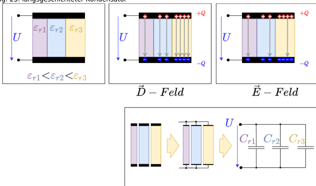
Fig. 23: längsgeschichteter Kondensator
