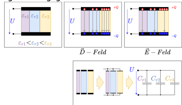
Fig. 23: längsgeschichteter Kondensator
