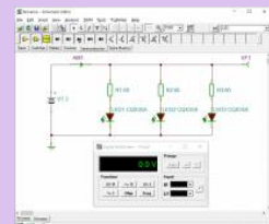
Fig. ##: Parallelschaltung 2
