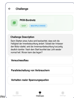
Mobile-Mockup...
