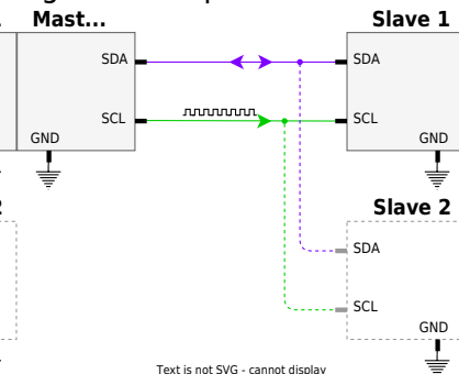
Fig. 3: Konzeptbild I2C
