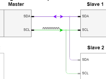
Fig. 3: Konzeptbild I2C
