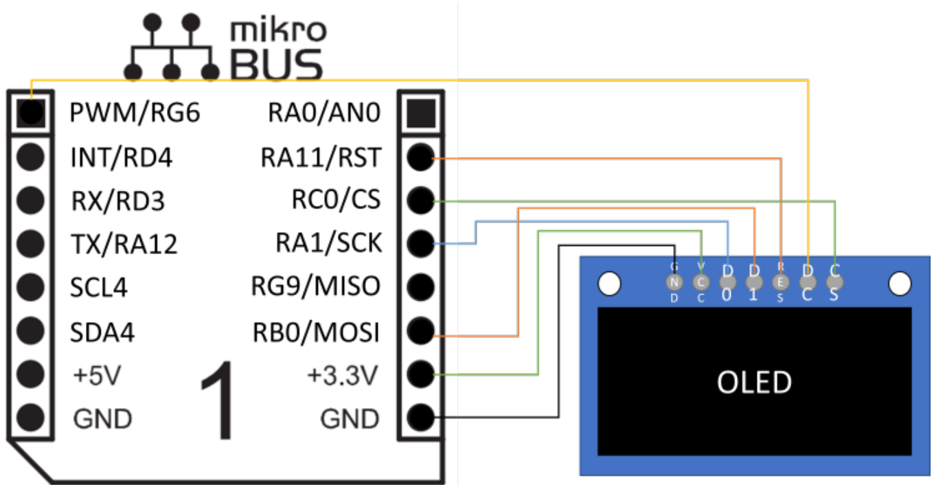
Fig. 32: Anschluss OLED
